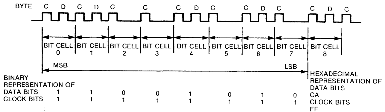
FIGURE 6-1. BYTE (FM ENCODING)
